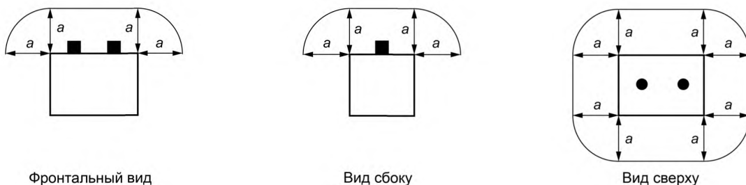
а) Аккумулятор с верхним расположением клемм
