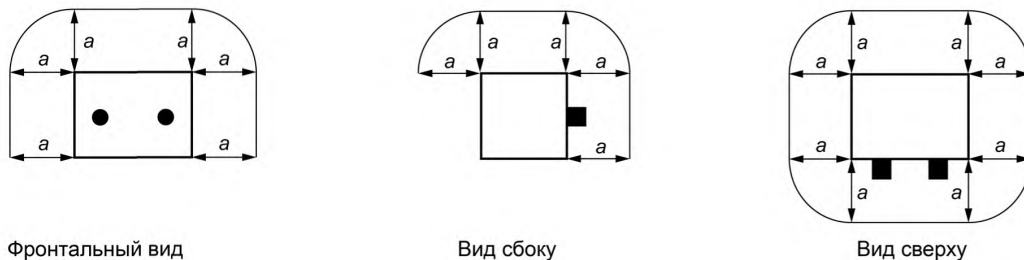
б) Аккумулятор с фронтальным расположением клемм
